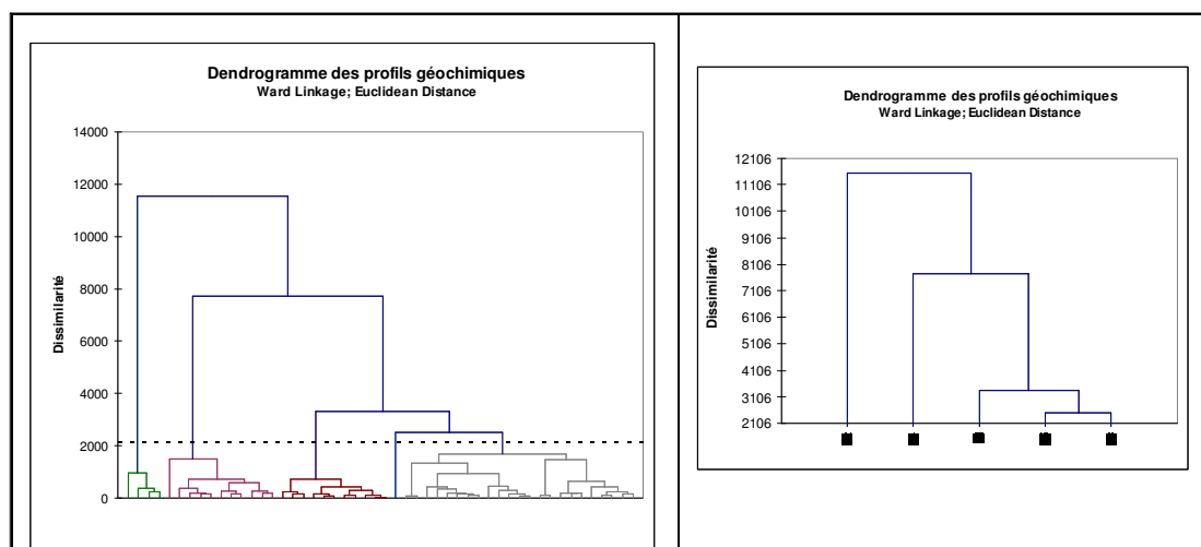
Figure 9. Dendrogramme des profils géochimiques
